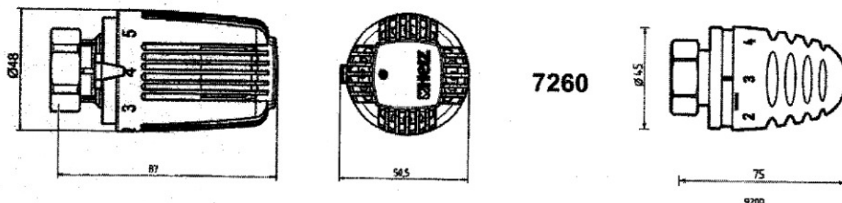
Slika 1. Izgled i dimenzije termostatskih glava STANDARD i MINI artikl br.7260 i 9200
